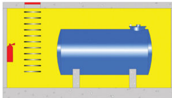
Tanque en fosa
