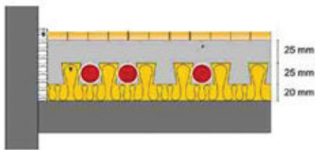
DETALES MONTAJE DE TUBOS CON PANEL AISLANTE MOLDEADO
